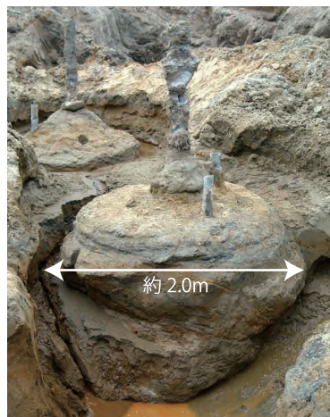
改良体出来形 (W/C=400%)
