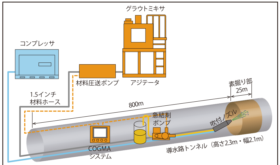
図-1 キロ・フケール工法の施工システム
